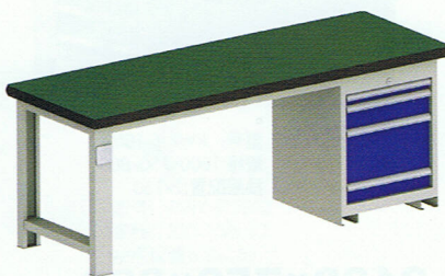
型号: RWK-F-2104 规格: 2100×750×800 抽屉配置: 2×75-1×150-1×250
