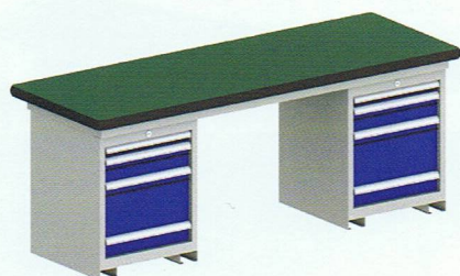
型号: RWK-2F-2104 规格: 2100×750×800 抽屉配置: 带2个RFL-06502工具柜
