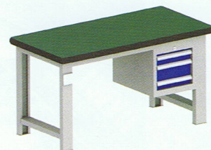
型号: RWK-S-1503 规格: 1500×750×800 抽屉配置: 2×75 1×150
