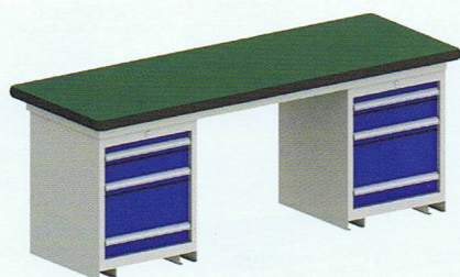
型号: RWK-2F-2105 规格: 2100×750×800 抽屉配置: 配2个RFL-06501工具柜
