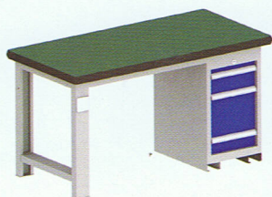
型号: RWK-S-1504 规格: 1500×750×800 抽屉配置: 1×100 1×150 1×300
