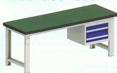
型号: RWK-F-2102 规格: 2100×750×800 抽屉配置: 2×150
