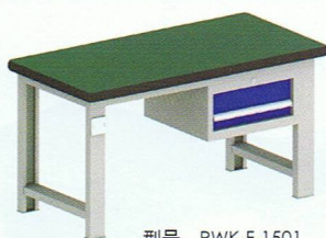
型号: RWK-F-1501 规格: 1500×750×800 抽屉配置: 1×200
